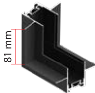
90° Dikey Bağlantı Aparatı Sıvaaltı 90° Vertical Joint Recessed ● Siyah/Black AD45-95000
